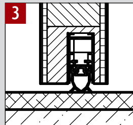
3 BODENDICHTUNG
